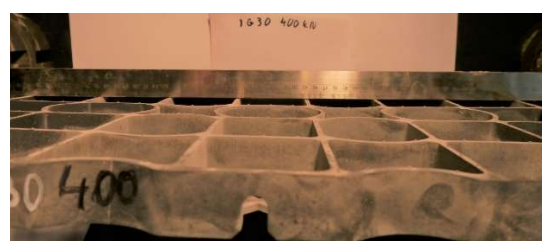
Fot. 6. Krata IG 30 400 kN
